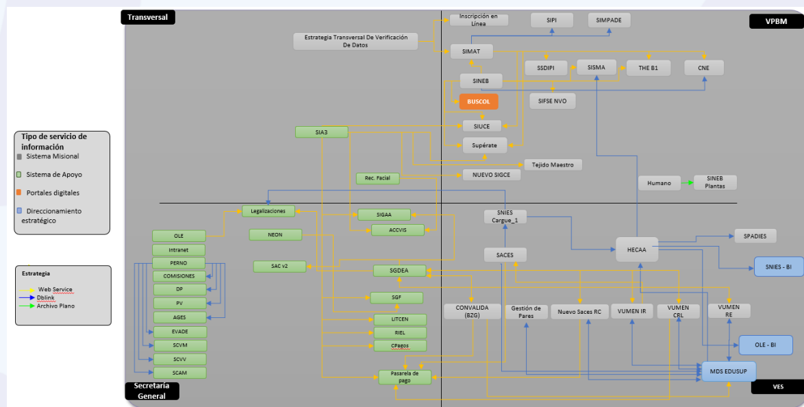
Ilustración 15. Servicios de información con estrategias de interoperabilidad interna
