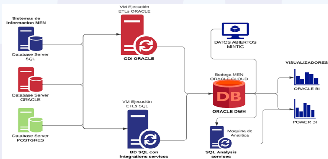
Ilustración 12. Diagrama de integración MinEducación S.I. con SQL – ORACLE
