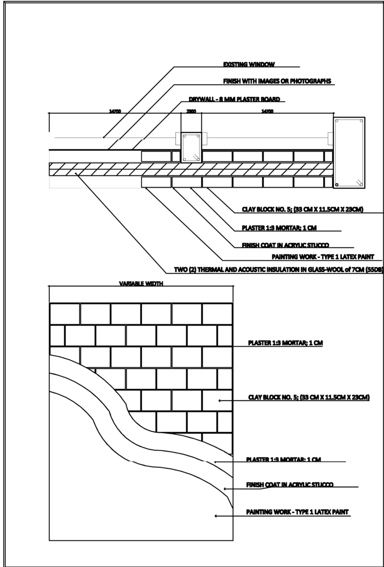
DET. 3
