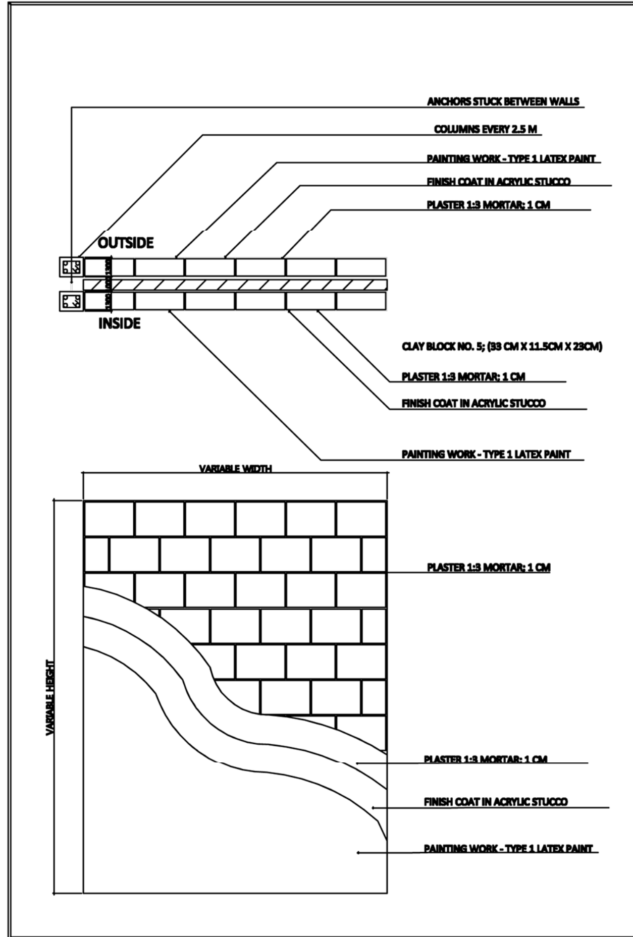
DET. 4
