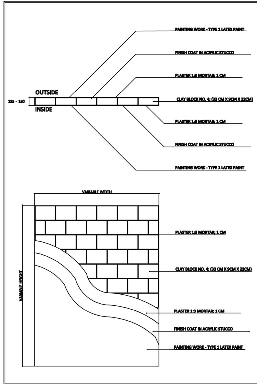
DET. 2
