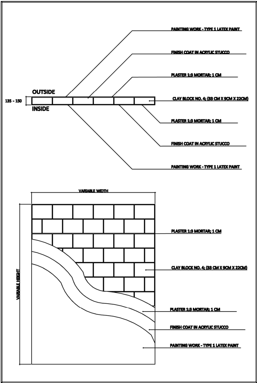
DET. 2
