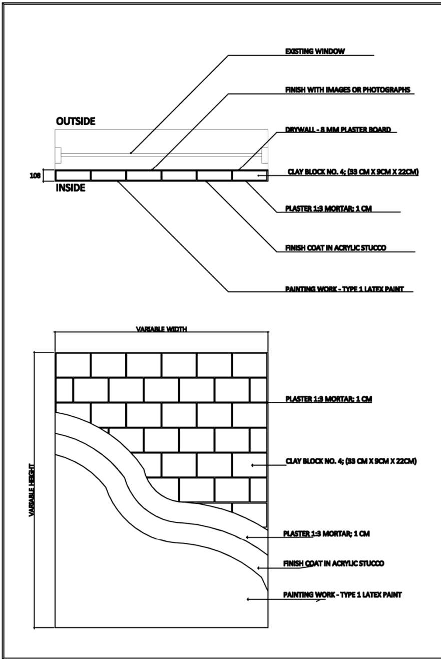
DET. 1
