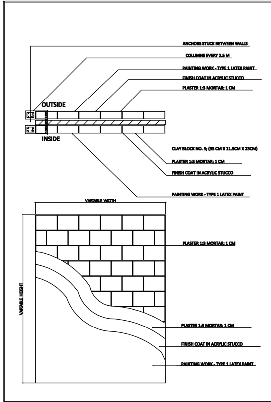
DET. 4
