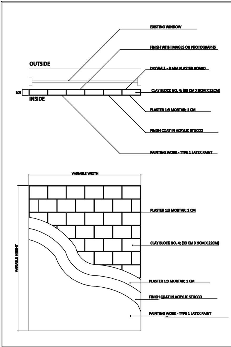
DET. 1
