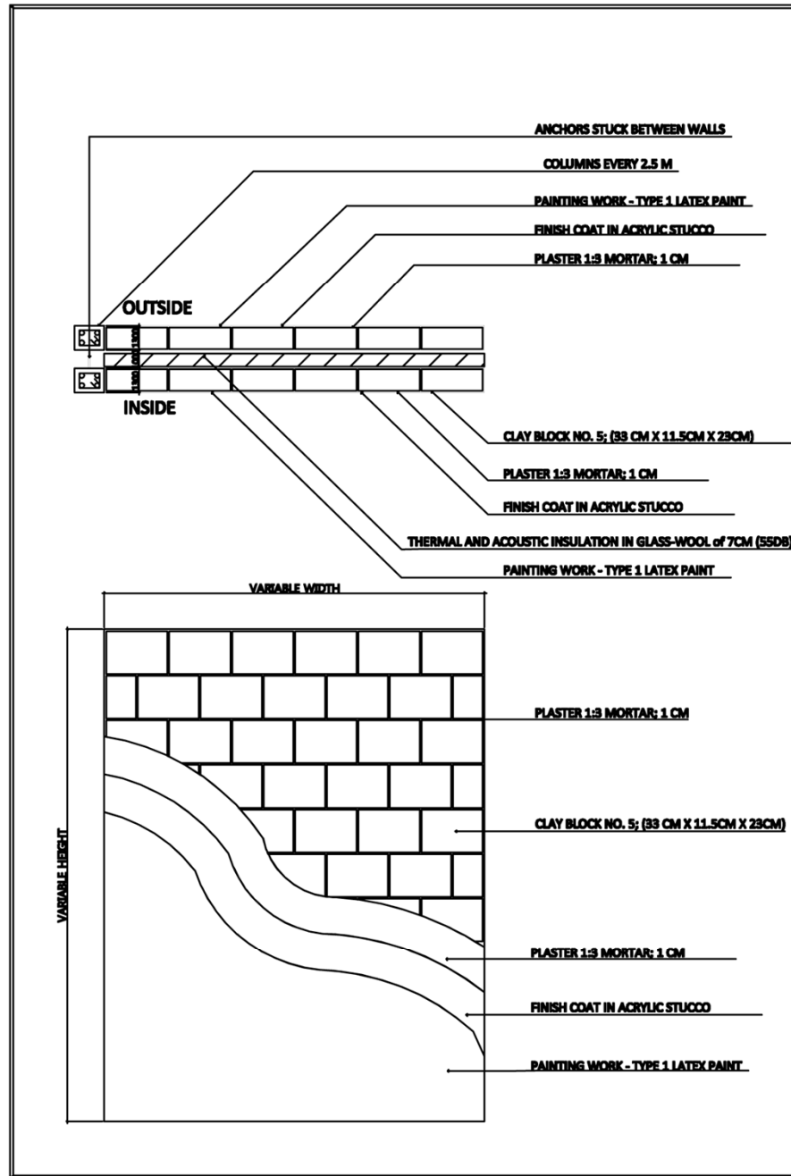
DET. 4
