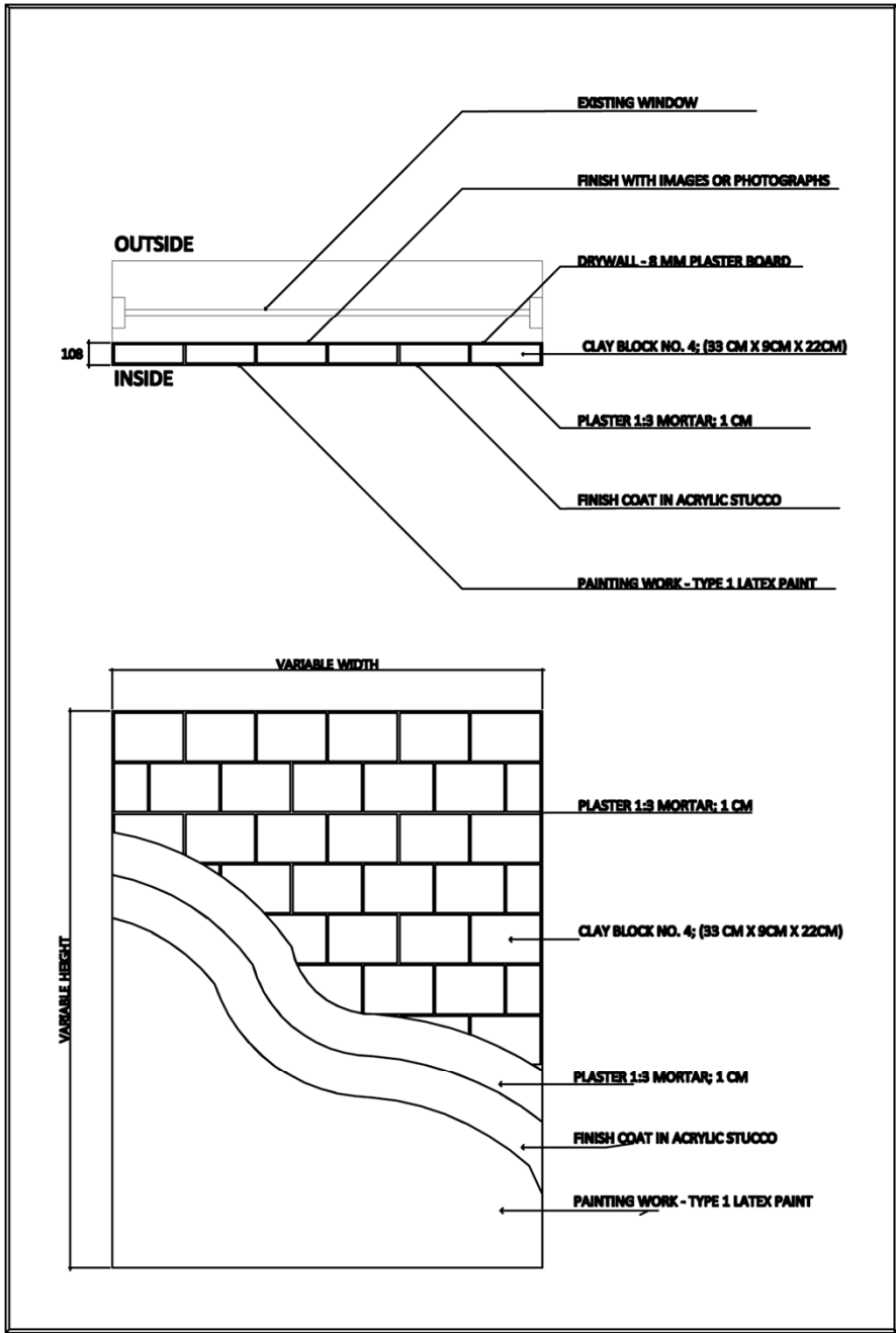
DET. 1
