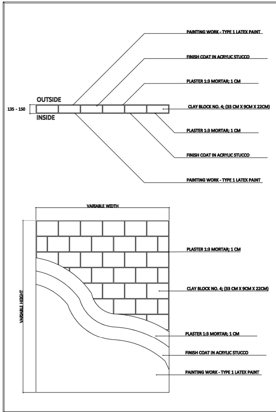
DET. 2
