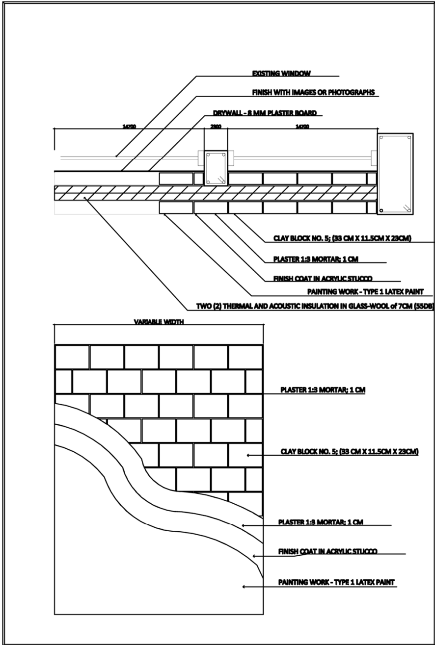
DET. 3
