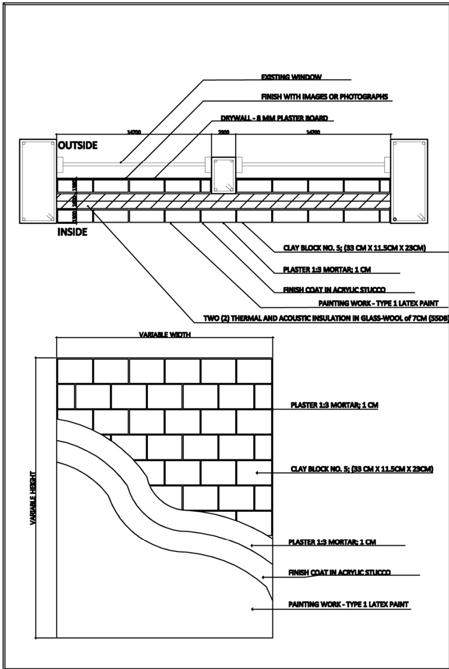
DET. 3
