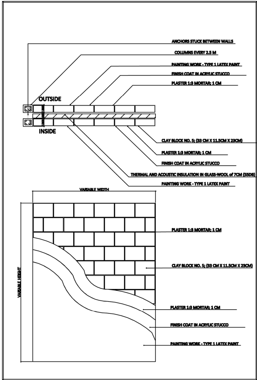
DET. 4
